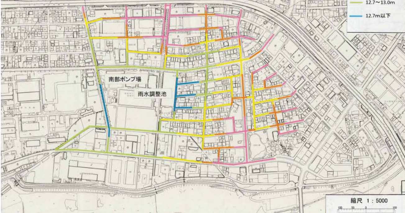
松河戸地区の雨水管路図
